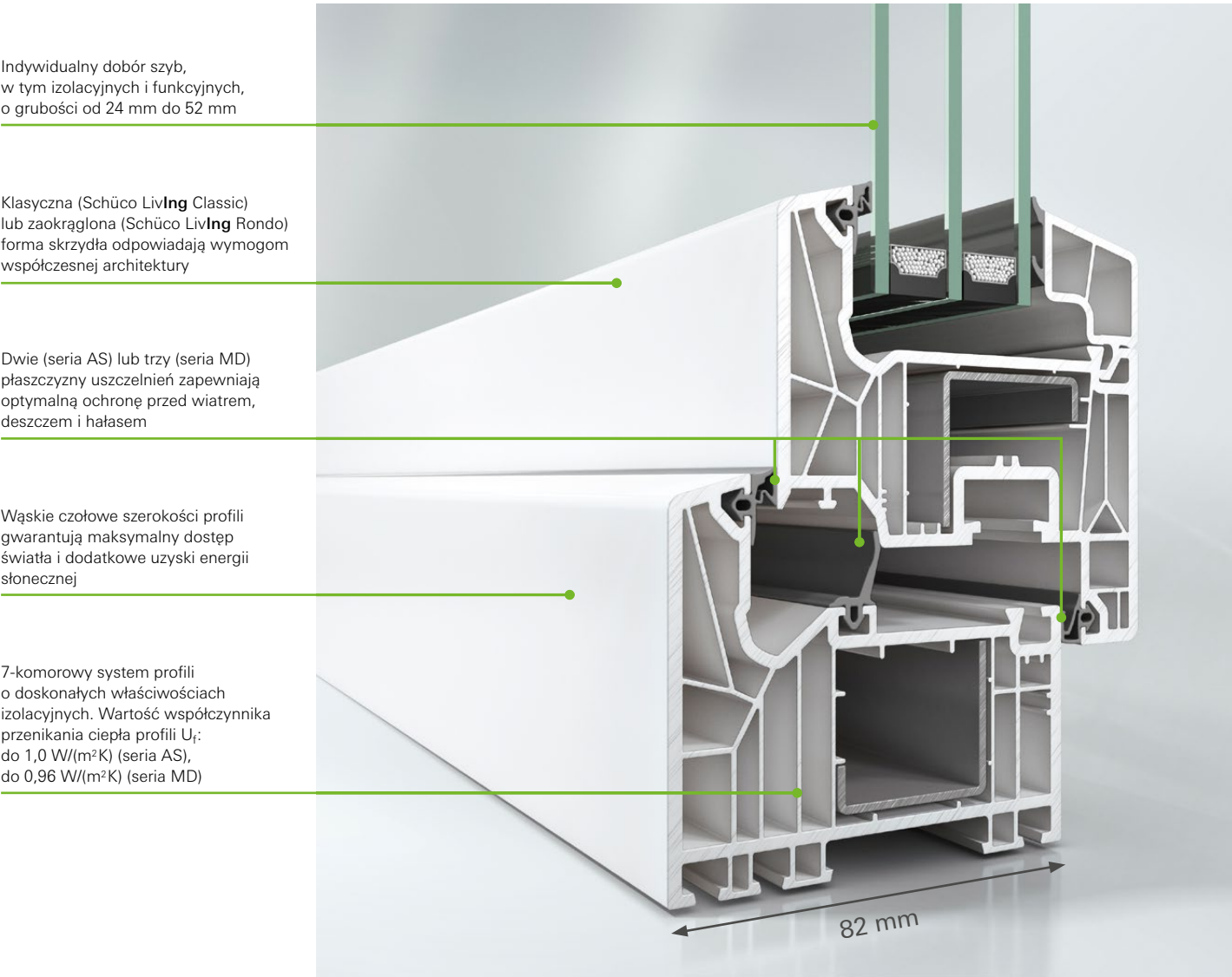
Schüco LivIng Classic 82 MD
