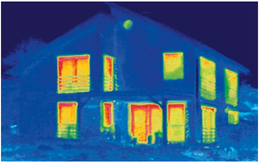
Zdjęcia termograficzne wyraźnie pokazują, w których miejscach energia cieplna wymyka się spod kontroli. Kolor czerwony to ciepło, a więc znacząca strata energii.
