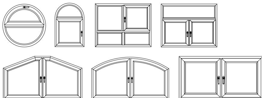
Wielodzielne okna i drzwi balkonowe
